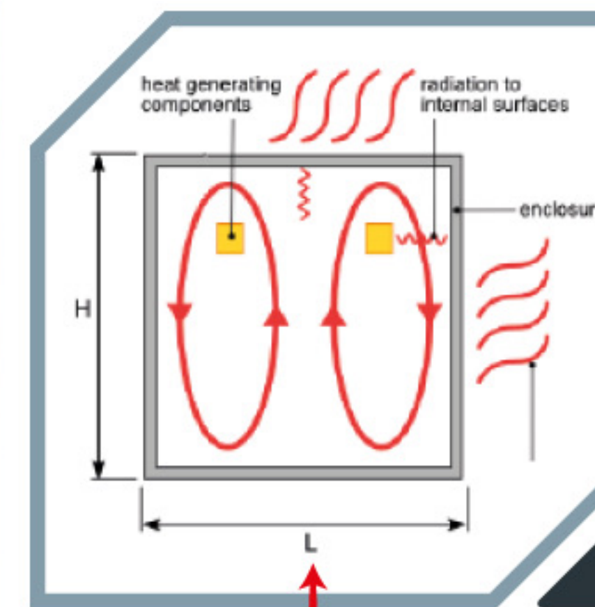
Enclosure without FAN
