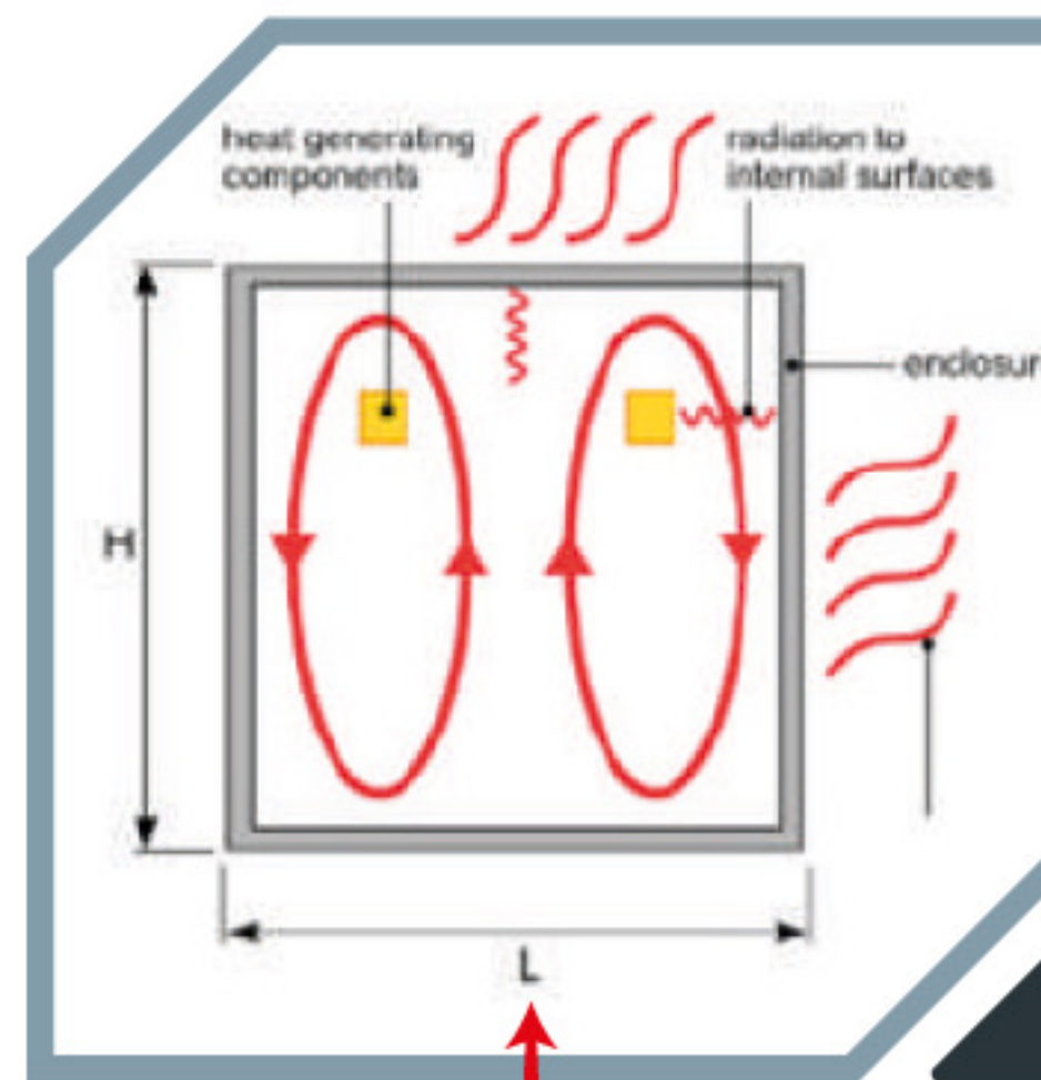
Enclosure without FAN
